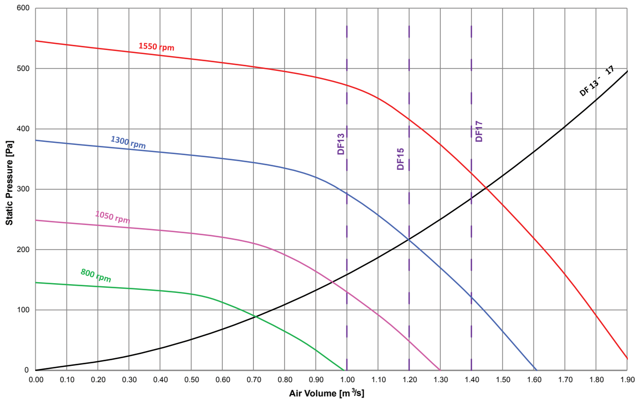
DF13- 17 EC Backward Fan Curve
