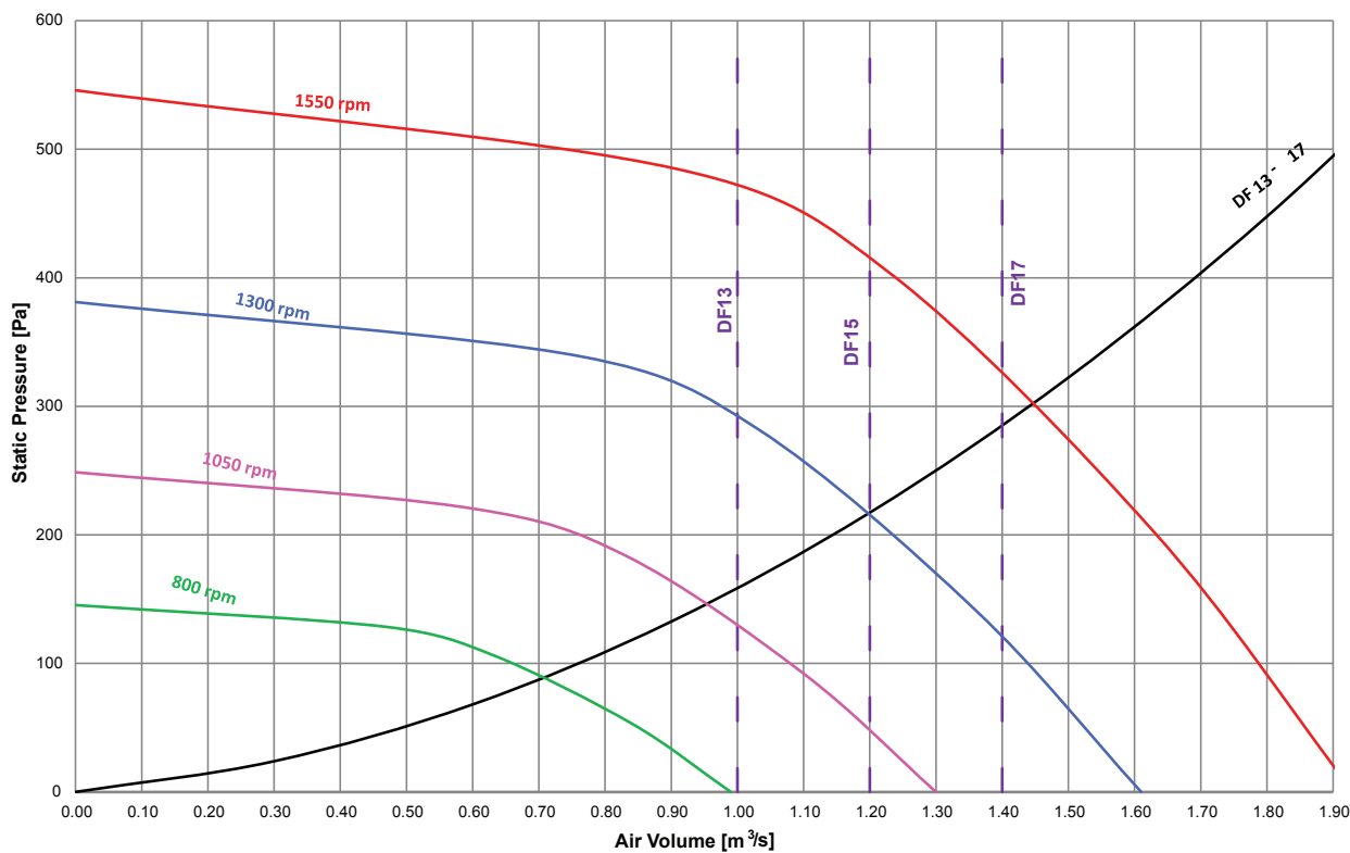
DF13- 17 EC Backward Fan Curve
