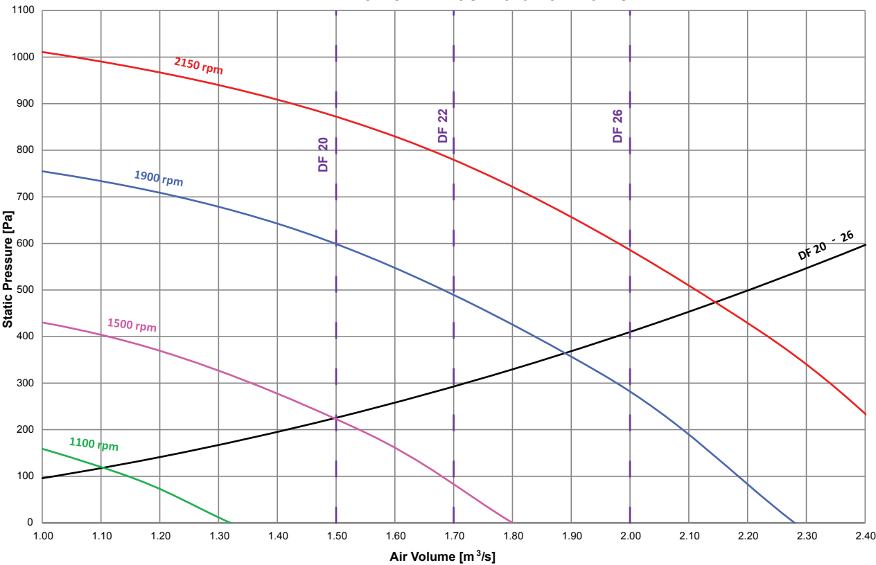
DF20- 26 EC Backward Fan Curve
